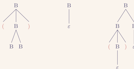
FIGURE 1 – Exemple d'arbres de dérivation
